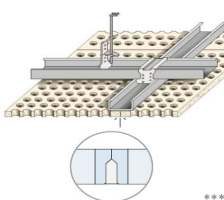
6/18 VB Absorbente Acústico CLASE C***
