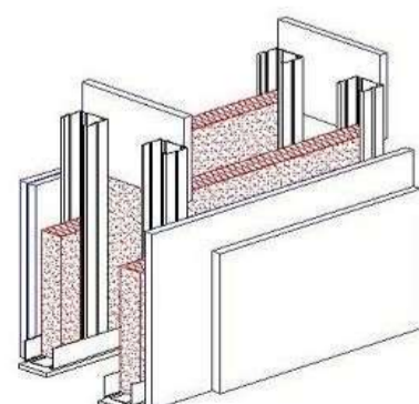
Tabique Multiple Doble Estructura
